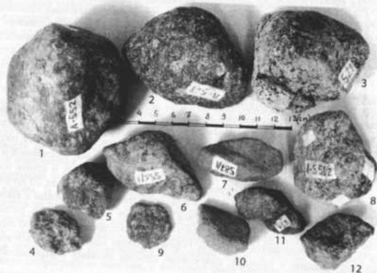
1-3 – бомбы округло-угловатой формы андезитов; 4, 5, 9 – лапилли лепешковидной формы андезитов-базальтов и базальтов; 7-7 – лапилли базальтов веретенообразной формы; 8, 10, 12 – лапилли базальтов изометричной формы; 11 – лапилли дацитов приплюснутой веретенообразной формы
