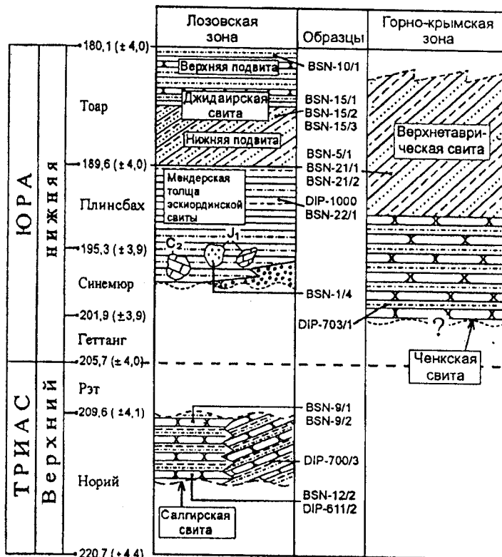
Рис. 1. Хроностратиграфическая схема расчленения триасовых и нижнеюрских отложений долины Бодрака [14]. Границы веков даны по [23]
