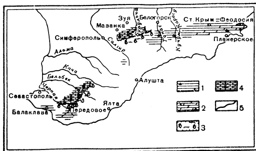
Рис. 1. Схема распространения гастропод в берриас-валанжинских отложениях Крыма: 1 — глины и 2 — мергели берриаса с Sulcoactaeon и Spinigera ; 3 — песчаники и алевролиты берриаса с Ampullina , Ampulospira , Scurgia и др.; 4 — гастроподовые известняки нижнего валанжина с Nerinea , Ptygmatis , Leviathania и др.; 5 — граница между берриасом и валанжином по полосе коренных выходов
