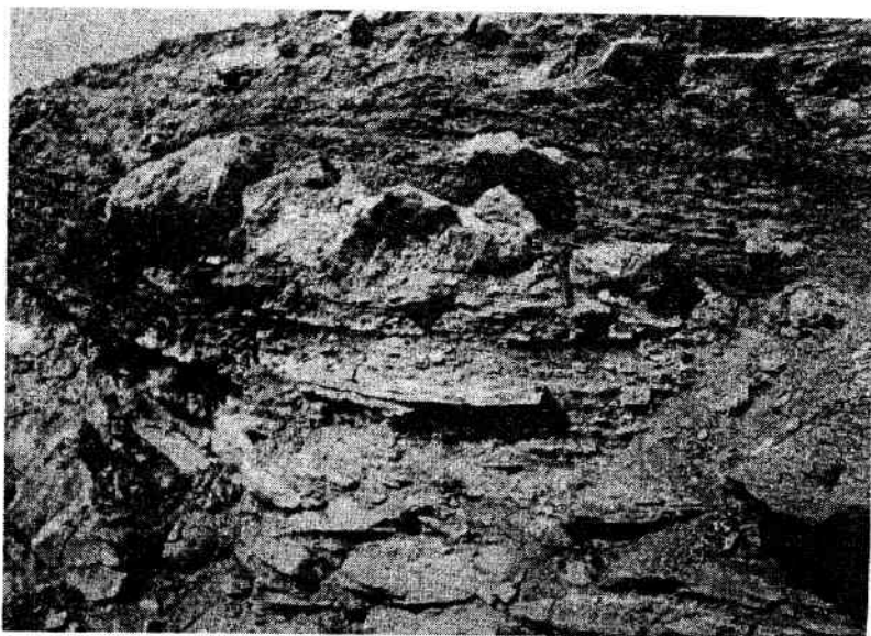
Рис. 2. Конгломератовая толща в глинистых алевролитах Нижняя граница резкая, дугообразной формы, с углублением вмещающих пород. Обнажение в нижней части старого Балаклавского карьера
