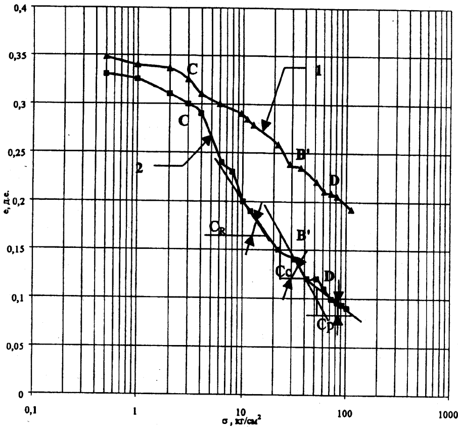
Рис. 3. Компрессионные кривые глин биязалинской свиты (K 1 br 2 -a): 1 — We = 14%; 2 — We = 15%
