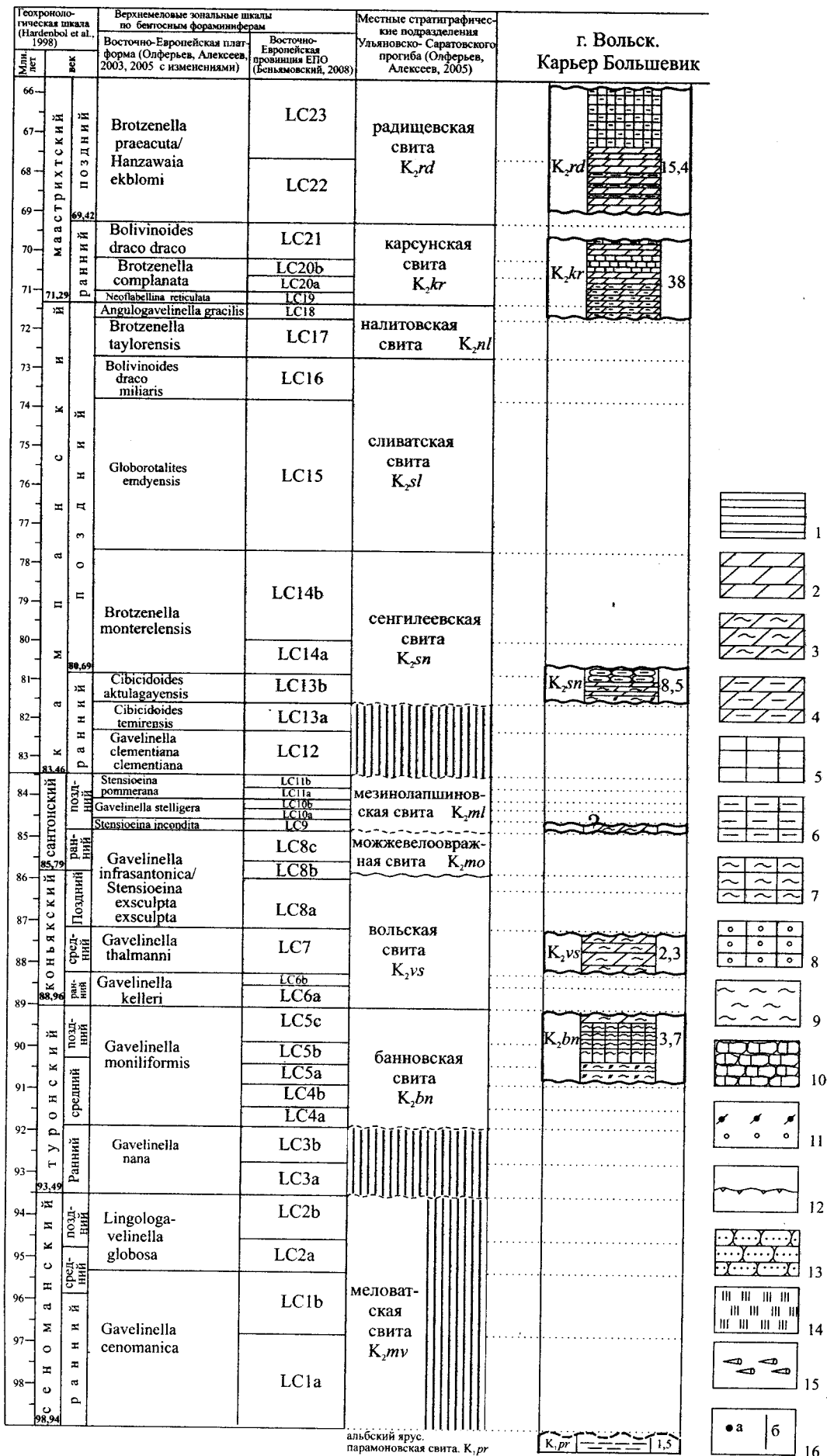
Рис. 9. Хроностратиграфическая схема строения верхнемеловых отложений района Вольска: 1 — глина; 2 — мергель; 3 — мергель алевроитистый; 4 — мергель глинистый; 5 — мел; 6 — мел глинистый; 7 — мел алевроитистый; 8 — мел с катунами известняка; 9 — алевроит; 10 — фазерный известняк; 11 — гравий и галька фосфорита; 12 — твердое дно; 13 — песчаник; 14 — опока; 15 — места находок белемнитов; 16 — места нахождения другой фауны: а — установленные, б — предполагаемые
