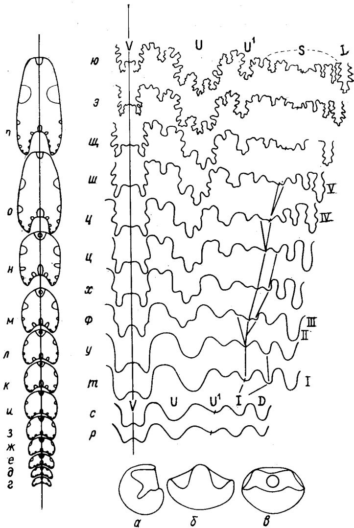
Рис. 5. Anahoplites rossicus Sinz.; а-в — начальная камера, экз. № 15374-III/151 (×33); г-п — изменение поперечного сечения в онтогенезе раковины; экз. № 14204/150: г — 3 перегородка (×10); д — 7 перегородка (×10); е — 9 перегородка (×12); ж — 14 перегородка, 1,2 об. (×10); з — 16 перегородка, 1,3 об. (×10,5); и — 19 перегородка, 1,7 об. (×9,5); к — 21 перегородка, 1,8 об. (×9,5); л — 24 перегородка, 2,2 об. (×9,0); м — 30 перегородка, 2,3 об. (×6); н — 34 перегородка, 2,7 об. (×5,5); о — 52 перегородка, к. 4 об. (×1,8); п — 68 перегородка, 4,7 об. (×1,2); р-ю — изменение лопастной линии в онтогенезе раковины; экз. № 8203/85: р — 4 линия (×41); с — 5 линия (×41); т — 11 линия, 1,3 об. (×41); у — 14 линия, 1,4 об. (×41); ф — 18 линия, н. 3 об. (×29); х — 22 линия, 2,2 об. (×24); ц — 26 линия, 2,5 об. (×20); ч — 30 линия, 2,7 об. (×18); ш — 36 линия, 3,2 об. (×12); щ — 41 линия, с. 4 об. (×8,3); э — 56 линия, 4,7 об. (×3,5); ю — 69 линия, н. 6 об. (×2); а-в — Мангышлак, Аксыртау, г-п — Мангышлак, Тюбеджик; р-ю — Мангышлак, Кугусем; верхний альб, зона A. rossicus
