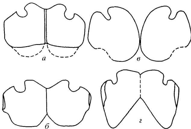
Рис. 2. Кораконды офталмосавринов: a – Vartanodon robustus (по Gilmore, 1906); б – Vartanodon discus (по Gilmore, 1905); в – Ophthalmosaurus icenicus (по Seeley, 1874); z – Paraophthalmosaurus saveljeviensis sp. nov.
