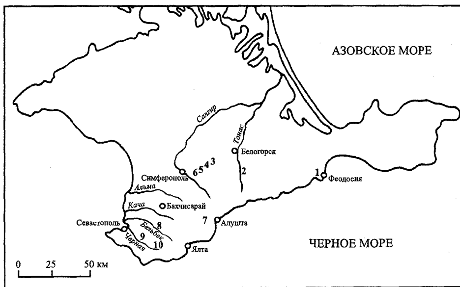
Рис. 1. Схема расположения изученных разрезов берриаса в Горном Крыму.
