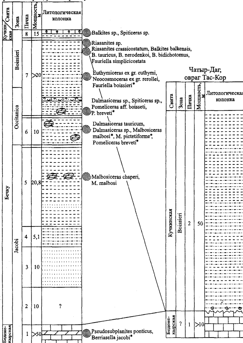
Рис. 5. Схема корреляции разрезов берриаса Центрального Крыма и массива Чатыр-Даг. Составил В.В. Аркадьев. Усл. обозначения см. на рис. 2. Знаком * отмечены виды, точная привязка которых к разрезу не совсем определенная.
