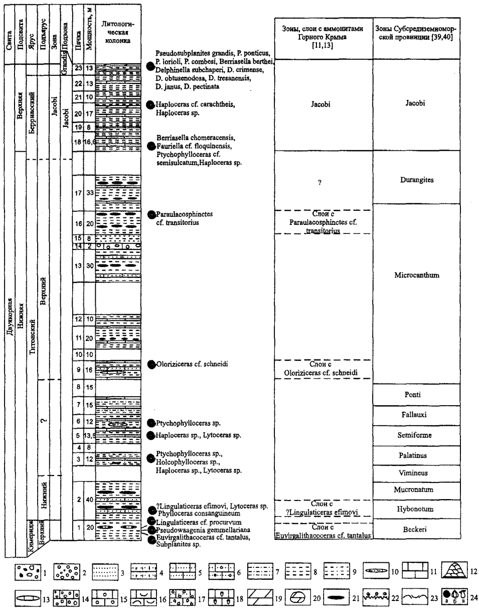
Рис. 2. Сводный разрез двукорной свиты Восточного Крыма по данным автора [11].
